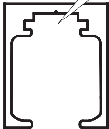
FD30-35EV 戸袋対応上レール (Pocket Door Type RAIL)
